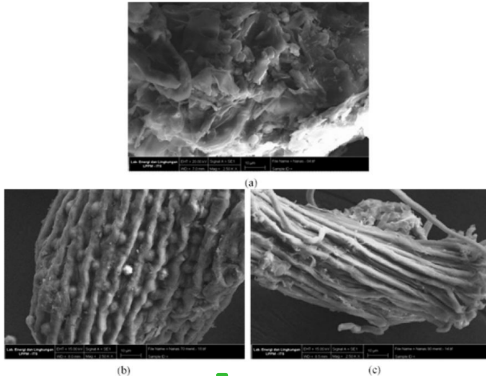
5 Gambar 4. Hasil Analisa SEM Perbesaran 2500x (a) Daun Nanas Sebelum Delignifikasi, (b) Daun Nanas dengan Delignifikasi 70 menit, dan (c) Daun Nanas dengan Delignifikasi 90 menit
