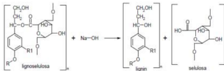
Gambar 2. Mekanisme Pemutusan Ikatan antara Lignin dan Selulosa Menggunakan NaOH (Zhang et.al, 2016)
