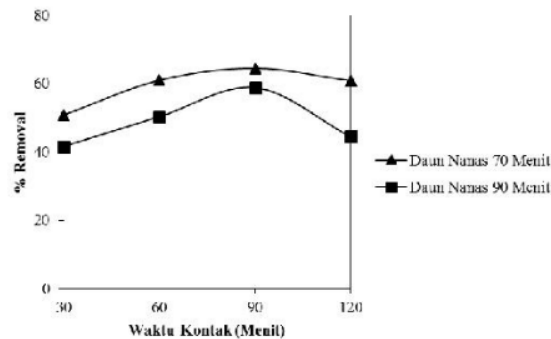
Gambar 5. Pengaruh Waktu Kontak terhadap Removal Logam Cu
