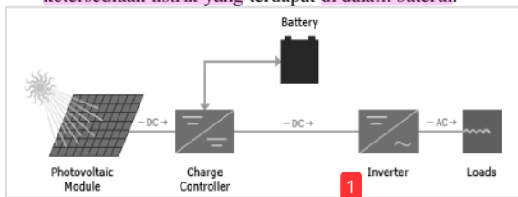
Gambar 1. Sistem PLTS Stand-Alone
