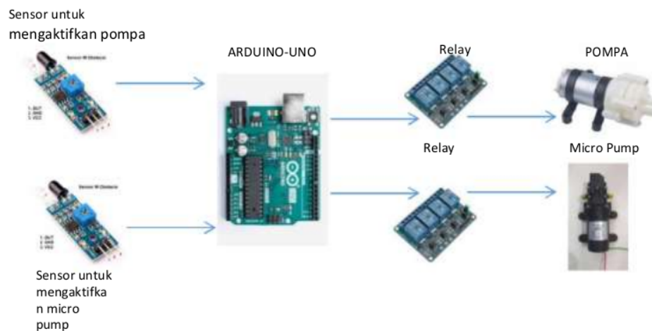
Gambar 2. Diagram Sistem Keseluruhan
