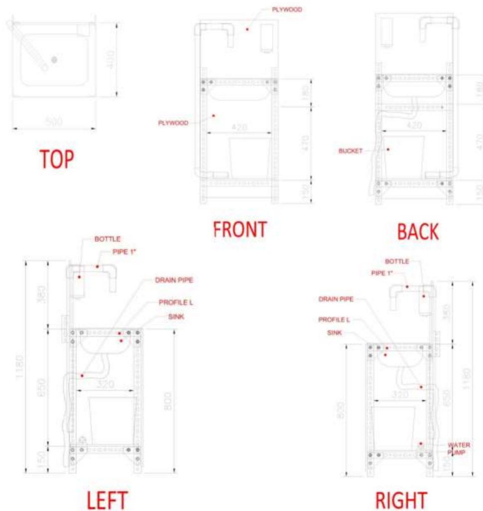
Gambar 3. Rancangan Tempat Pencuci Tangan
