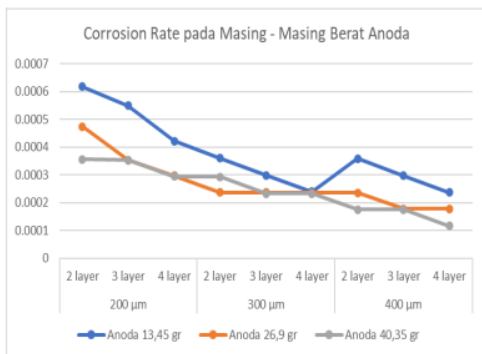
Gambar 4 Corrosion Rate pada Masing Masing Berat Anoda
