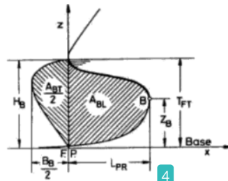
Gambar 2 Parameter desain bulbous bow
