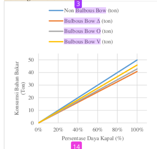
Gambar 6. Grafik Konsumsi Bahan Bakar
