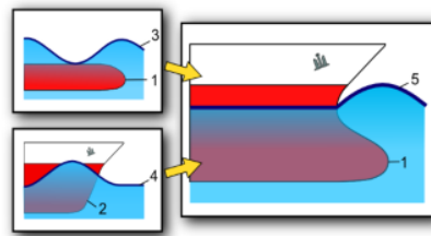
Gambar 1. Pengaruh gelombang bulbous bow
