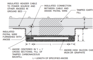
Gambar 3. Ilustrasi Pemasangan Horizontal Groundbed
