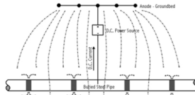
Gambar 1. Skema Proteksi Katodik ICCP
