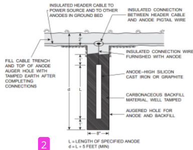
Gambar 2. Ilustrasi Pemasangan Vertical Groundbed
