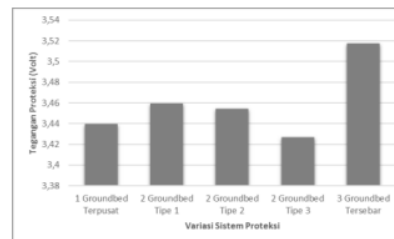
Gambar 5. Perbandingan Teknis Variasi Peletakan Groundbed
