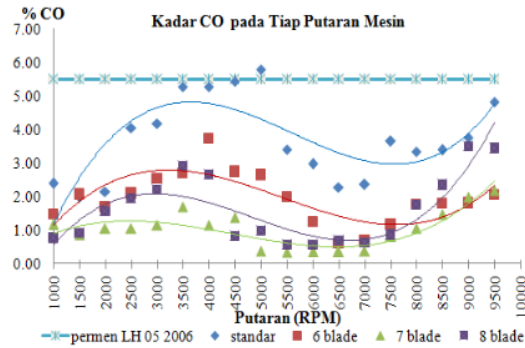
Gambar 2. Grafik perubahan kadar CO terhadap putaran mesin.
