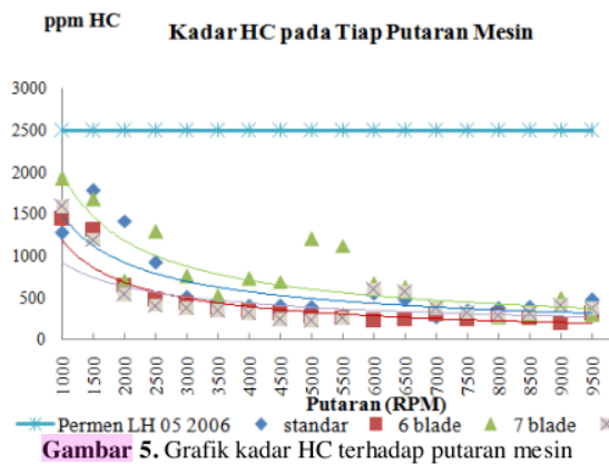
Gambar 5. Grafik kadar HC terhadap putaran mesin
